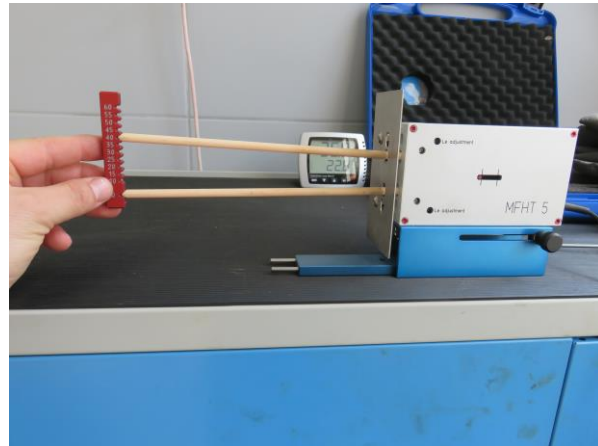
Određivanje merne dužine na ekstenziometru, fot. 2
